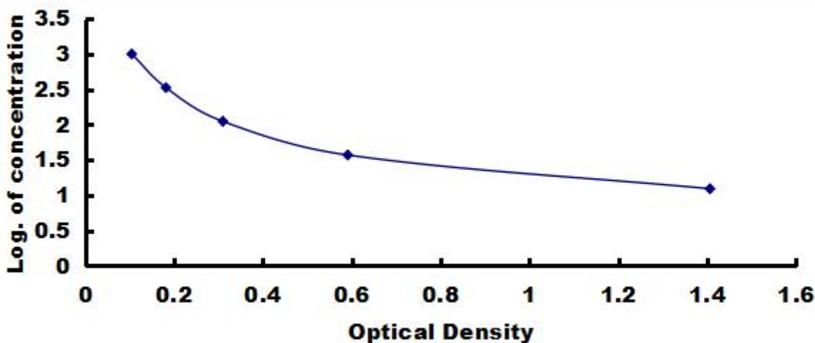
大鼠激活素 A (ACVA) 检测试剂盒标准曲线
