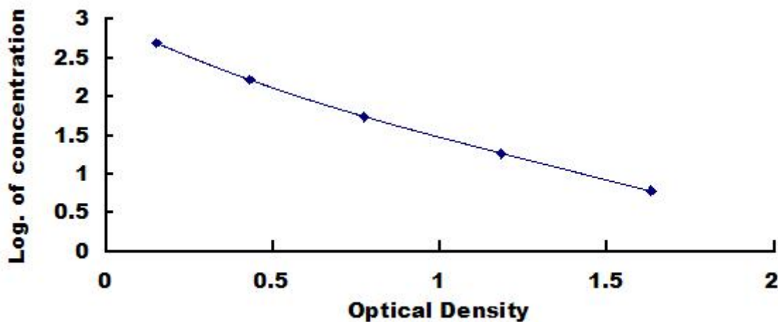
鞘氨醇(Sph)检测试剂盒标准曲线
