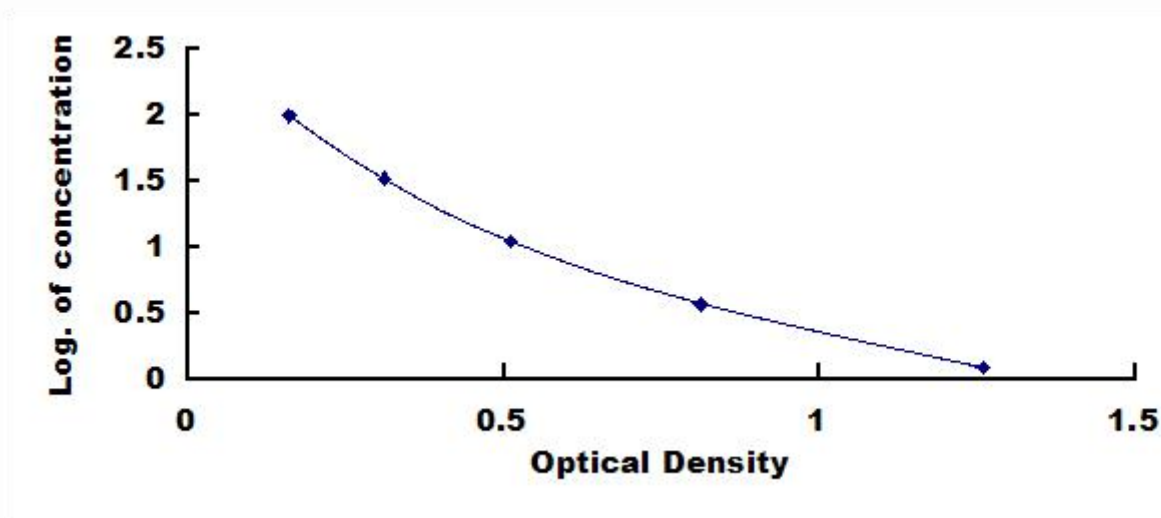
色氨酸(Trp)检测试剂盒标准曲线
